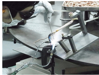
ロウ接加工
