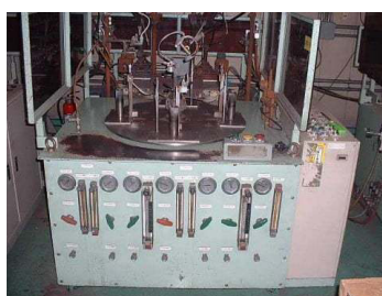
自動ロウ接装置
